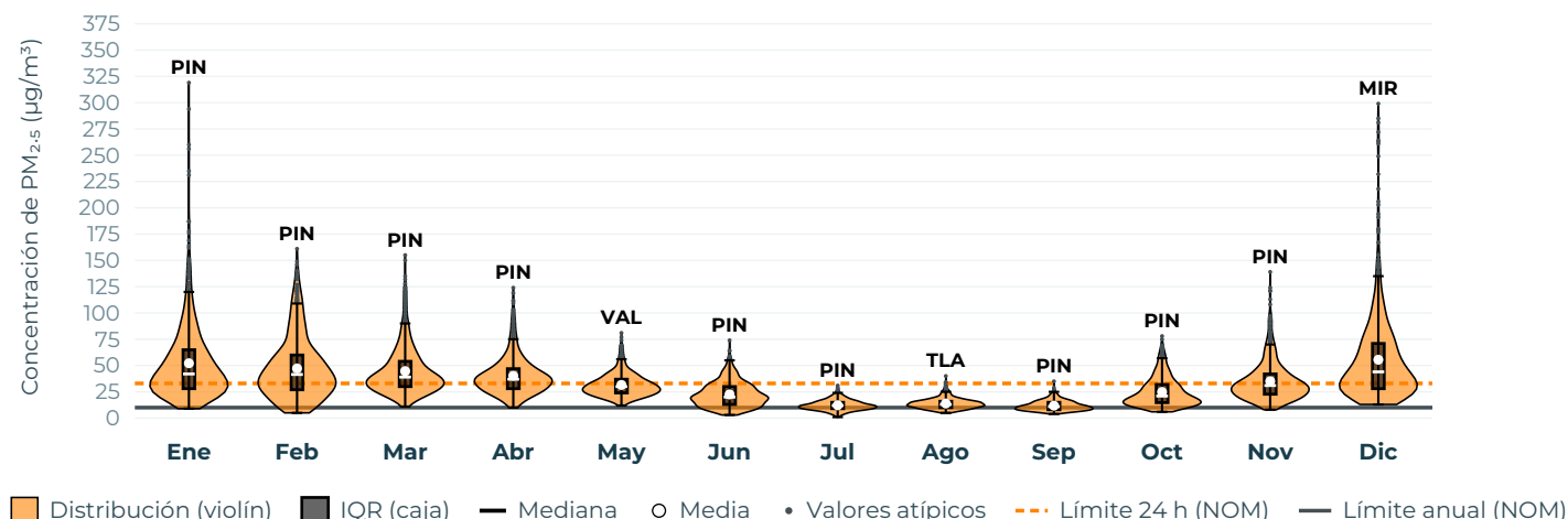
Figura 15. Distribución horaria mensual de PM 2.5 (NowCast, promedio ponderado de 12 horas) en el AMG, 2024.
