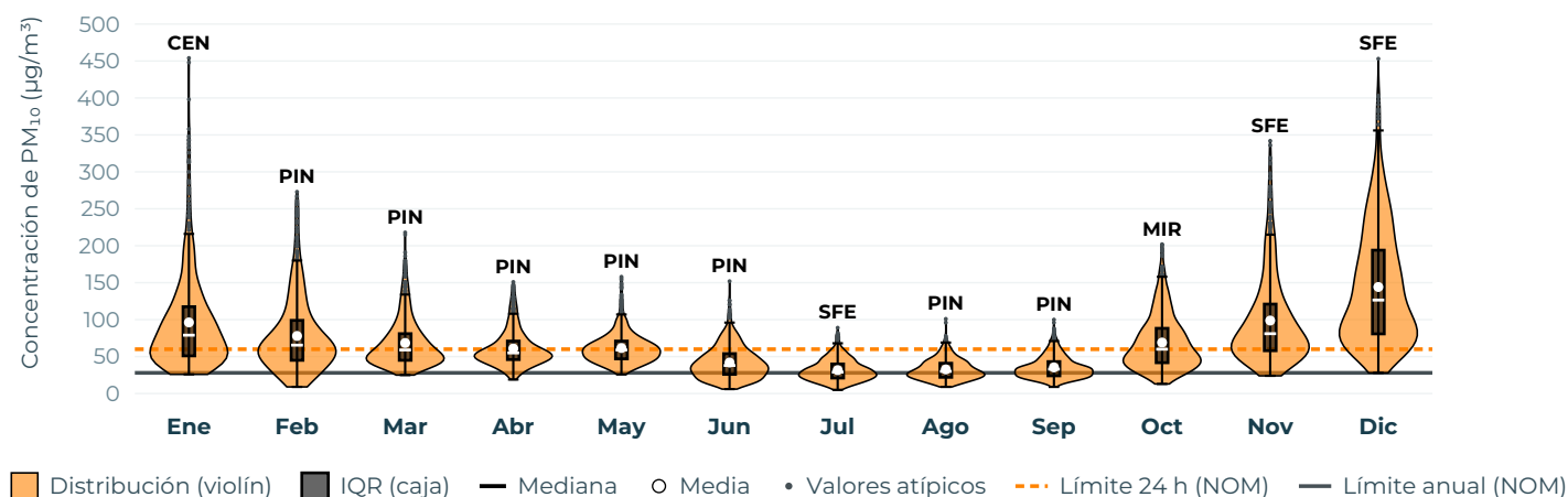
Figura 12. Distribución horaria mensual de PM 10 (NowCast, promedio ponderado de 12 horas) en el AMG, 2024.
