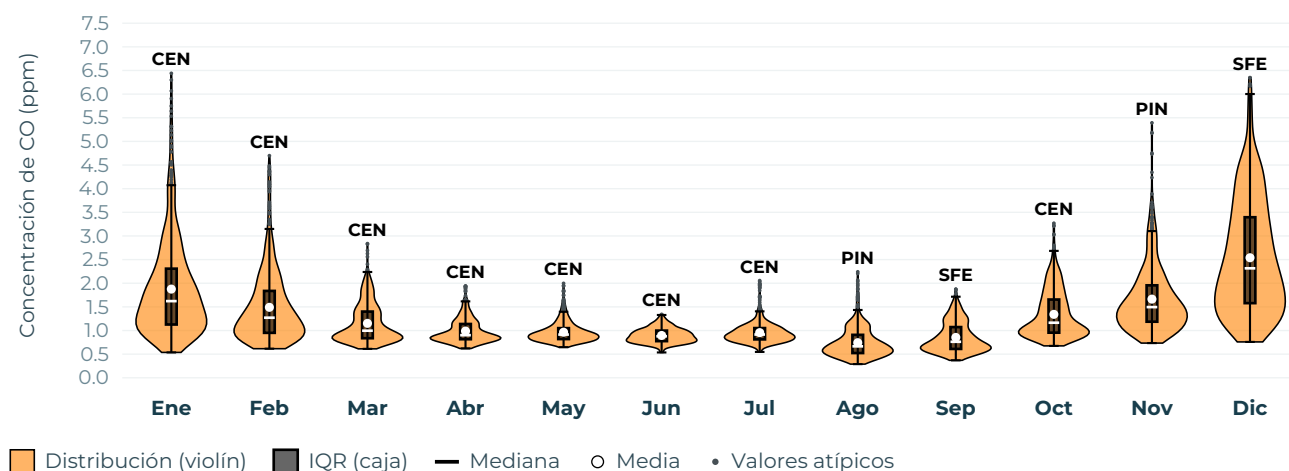
Figura 6. Distribución horaria mensual de CO (promedio móvil de 8 horas) en el AMG, 2024.
